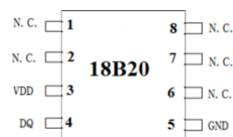
SOP8
