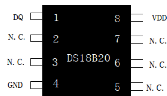
MSOP8
